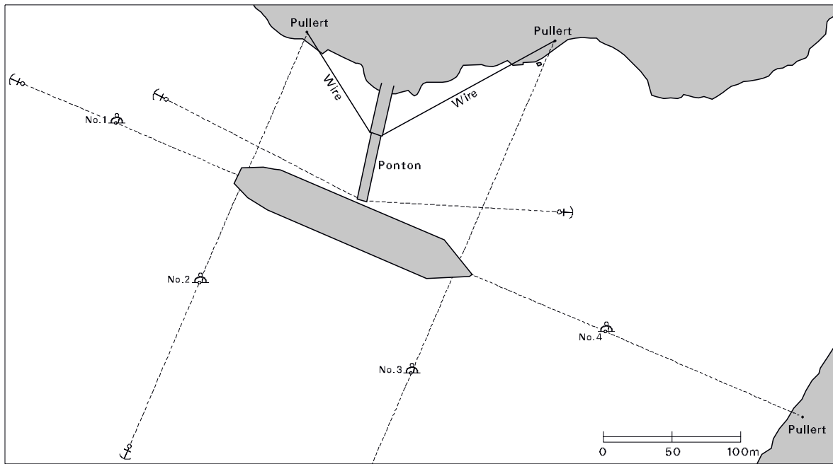
Skitse af Seqi Olivine A/S udskibningsanlæg
